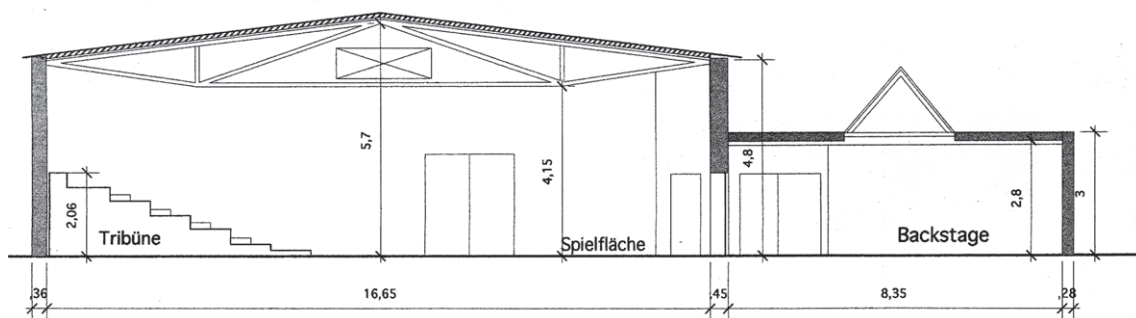
Schnitt M1:100
