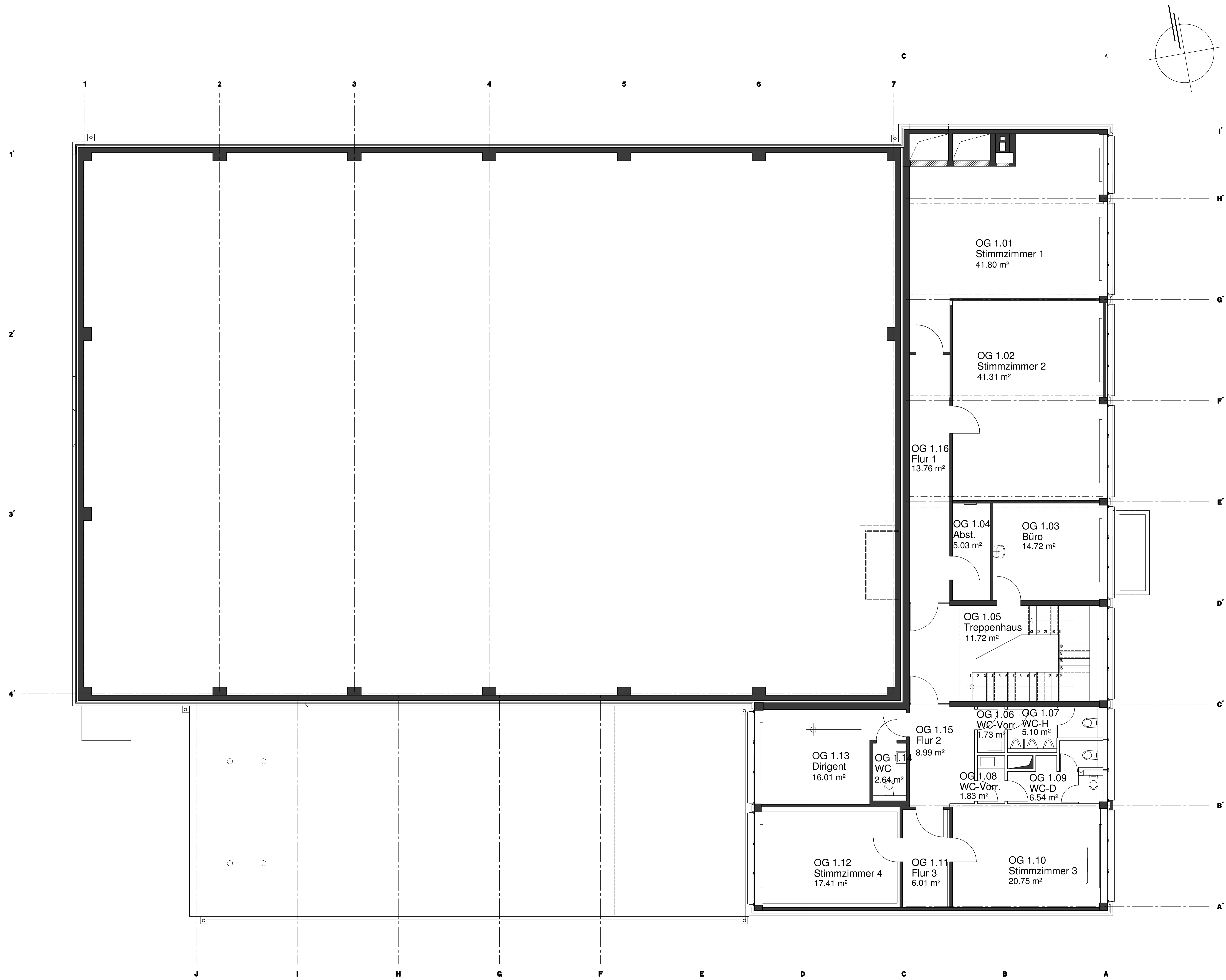
1. Obergeschoss
