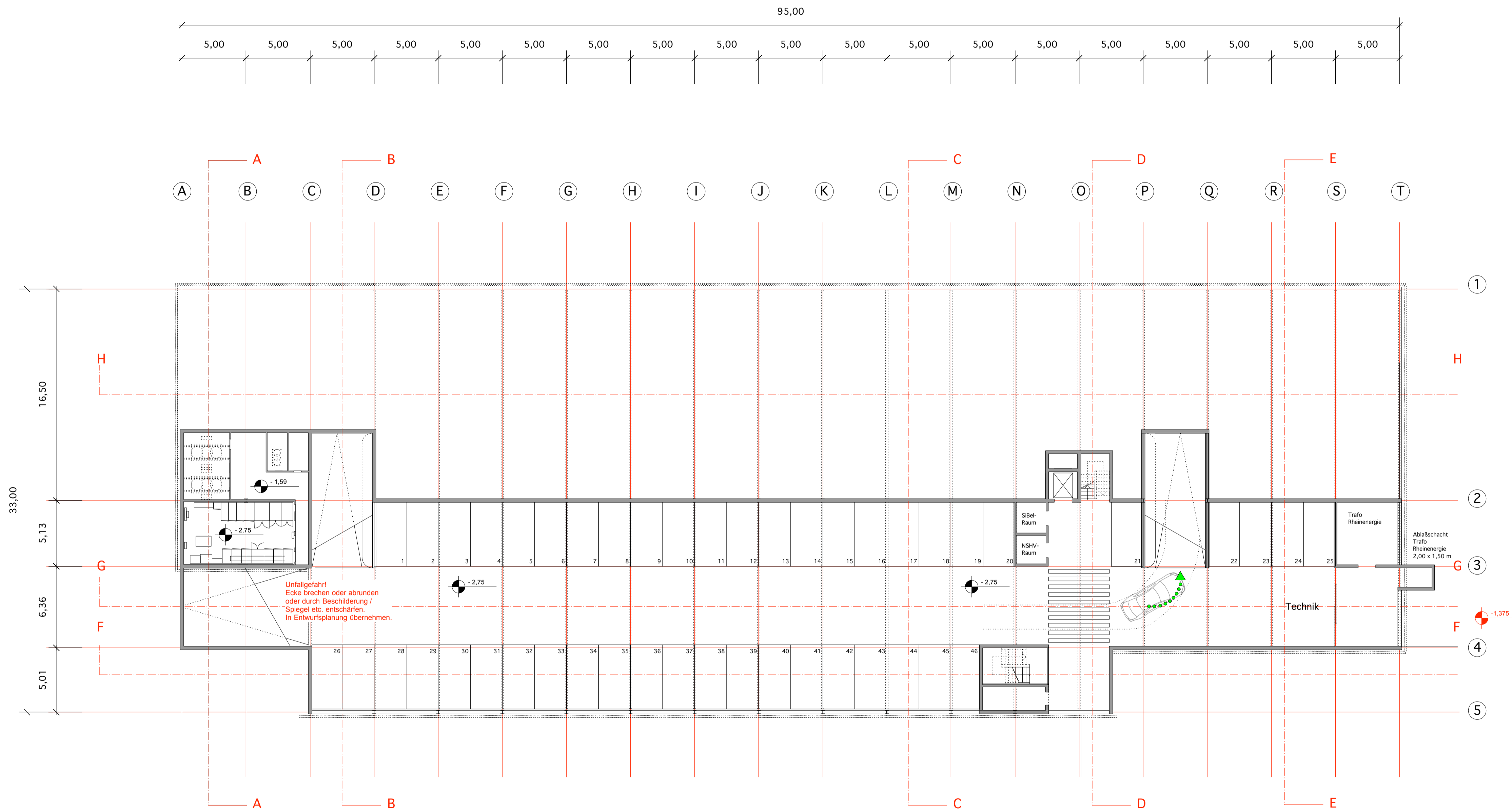
Grundriss Untergeschoss M 1:200
