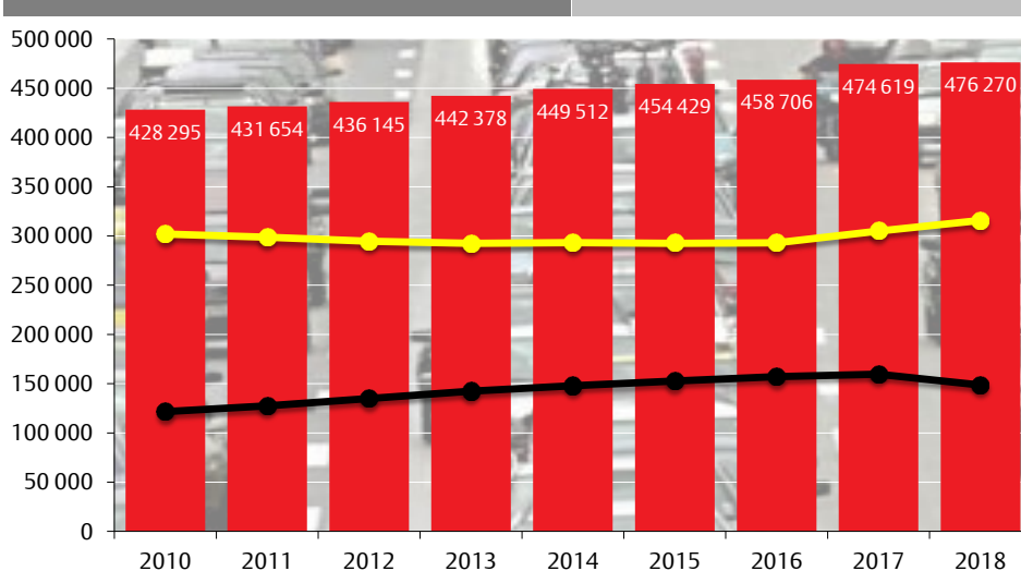
Kölner Pkw 2010-2018
