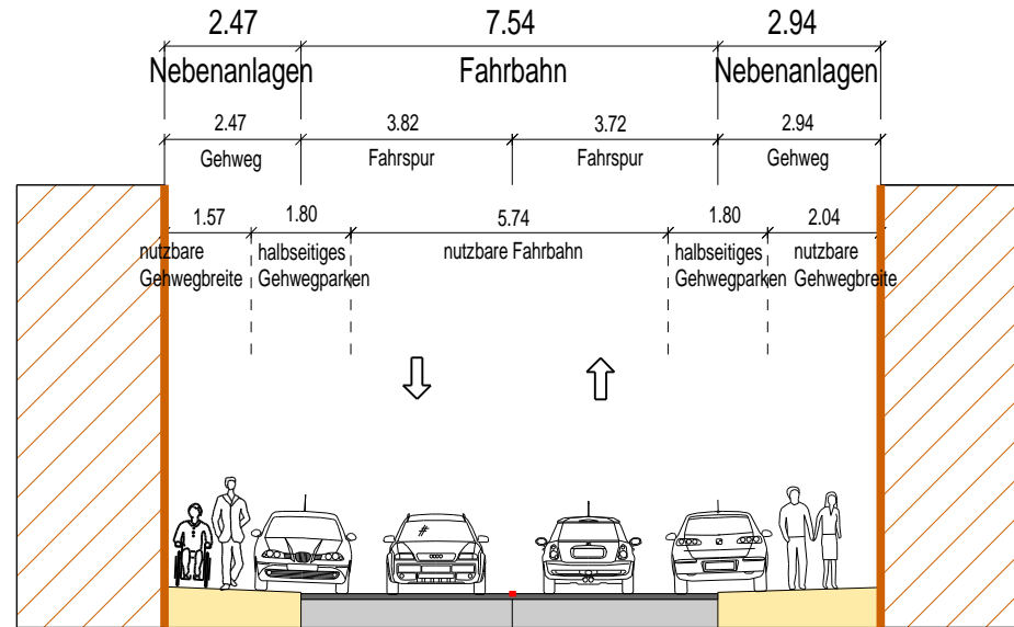
BESTAND Querschnitt A-A
