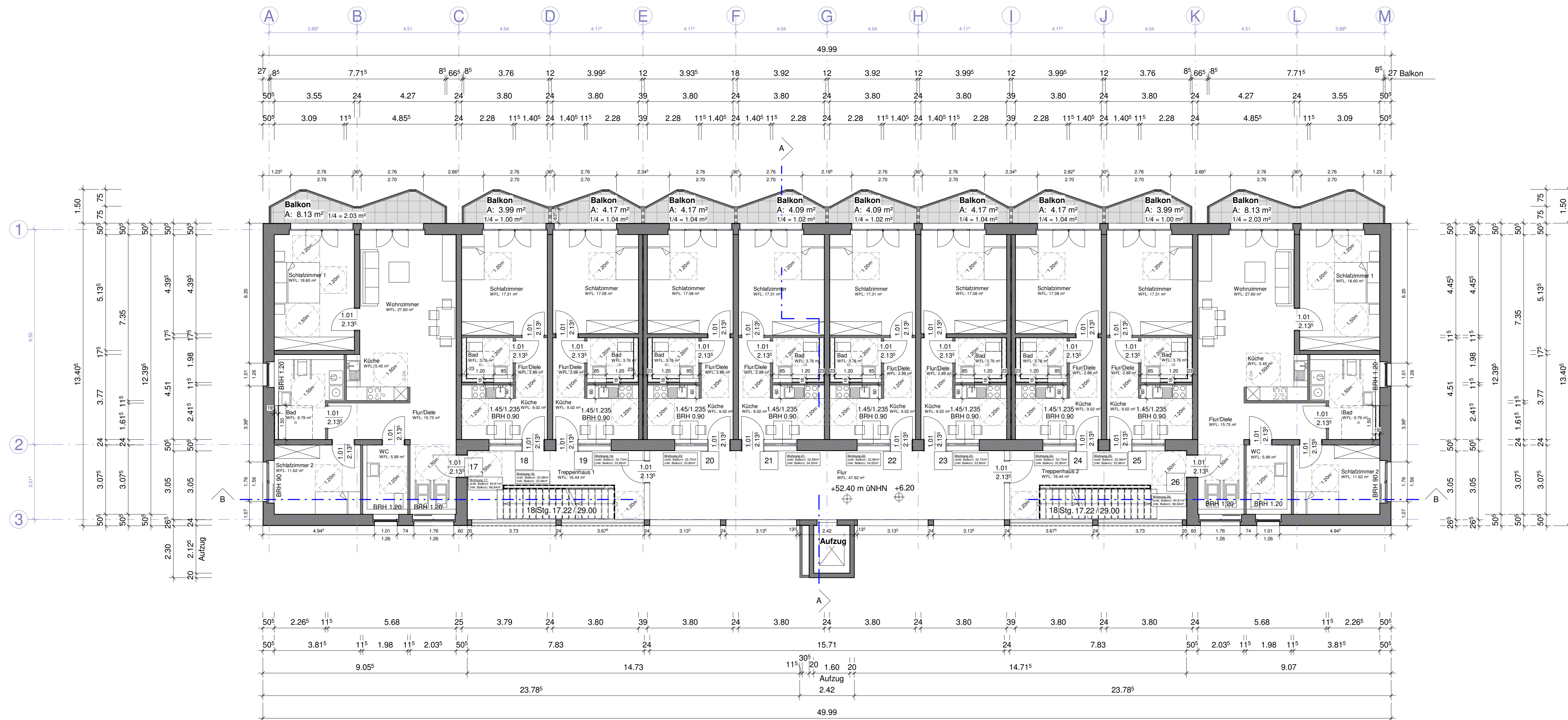
2.Obergeschoss
