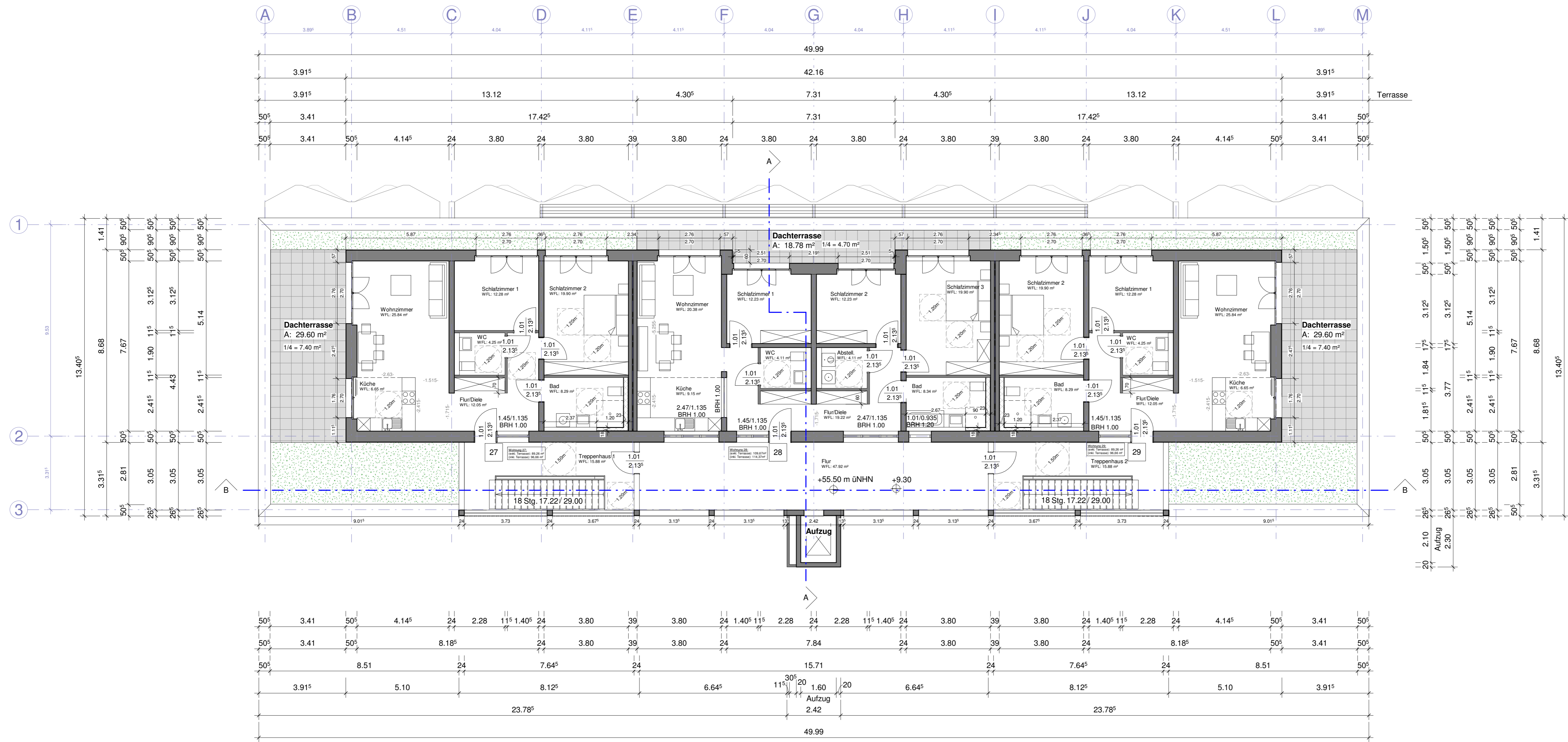
Dachgeschoss
