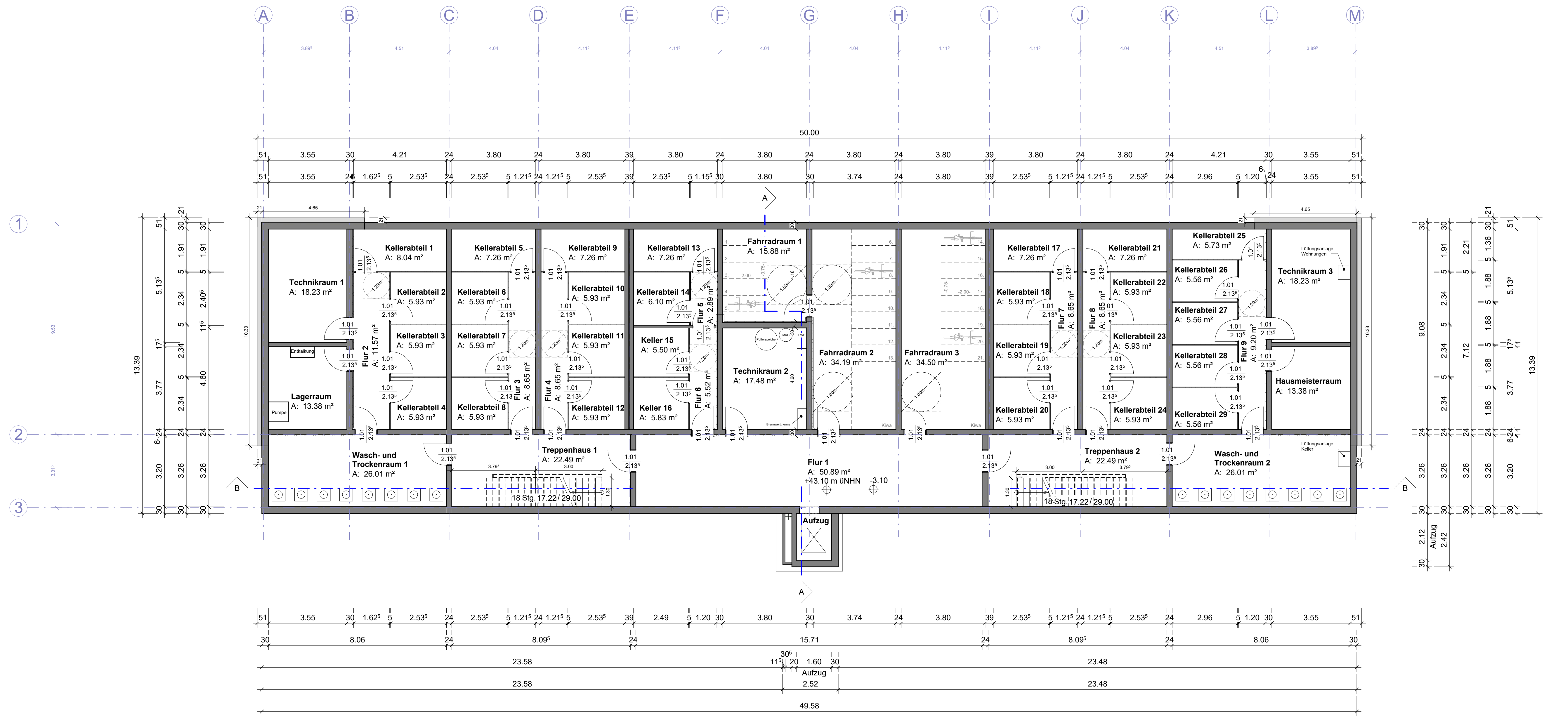
Untergeschoss
