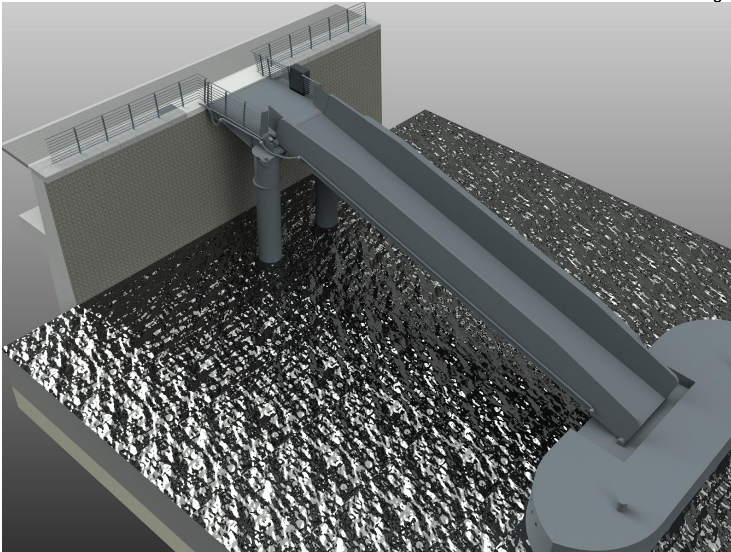
Isometrie Anlegestelle 0
