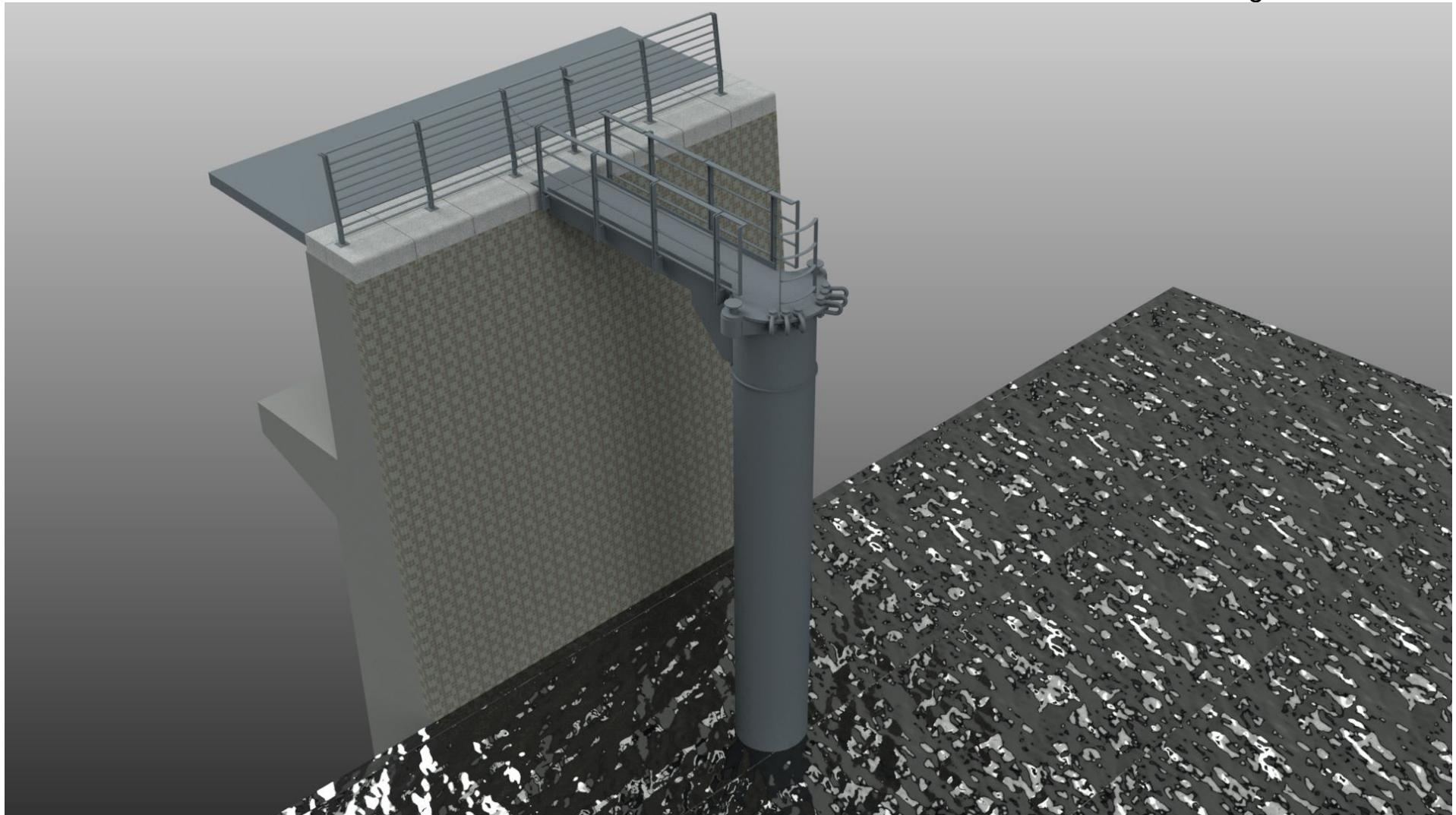
Isometrie Vertäudalben
